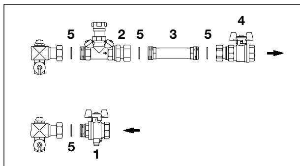
Fig. 2: Set di collegamento contacalorie, versione dritto, fornitura e montaggio dei componenti su lato dx.
