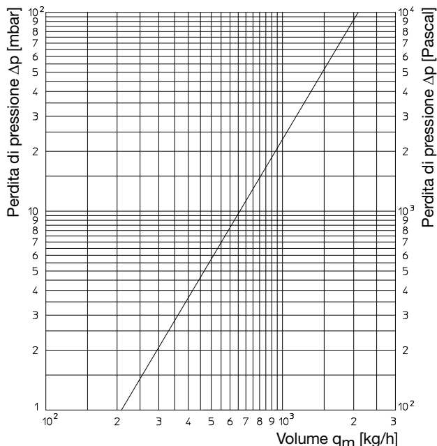
Diagramma 1: Perdita di pressione del set 1 di collegamento contacalorie
