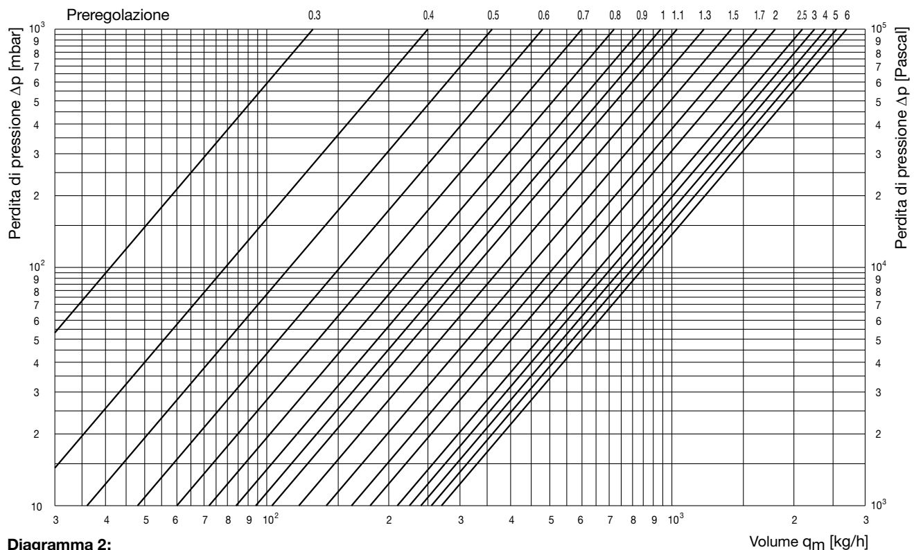
Diagramma 2: Perdita di pressione valvola di bilanciamento „Hycocn VTZ” DN 20
