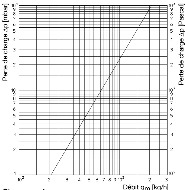
Diagramme 1: Perte de charge jeu de raccordement no. 1 pour compteurs de calories
