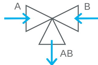
Utilizare ca ventil de amestec: debitul A și B sunt amestecate la ieșirea AB în funcție de cursa ventilului.
