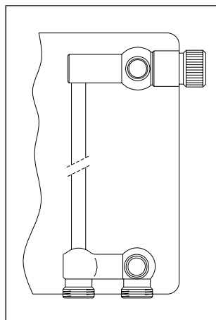
Radiator met geïntegreerd ventielgarnituur \frac{3}{4} " buitendraad, buisafstand 50 mm
