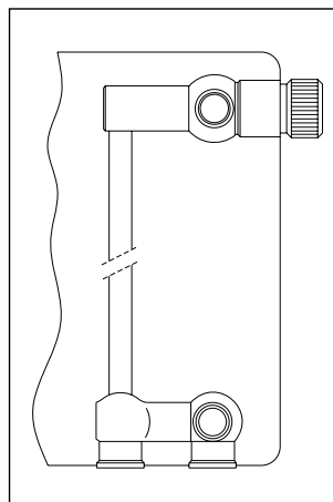
Radiator met geïntegreerd ventielgarnituur \frac{1}{2} " binnendraad, buisafstand 50 mm
