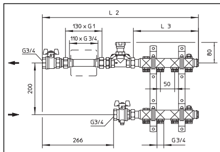
Fig. 2: set di collegamento per contacalorie- Set 1, diritto, con collettore inox „Multidis SH“ per il collegamento al radiatore, lunghezze e profondità
