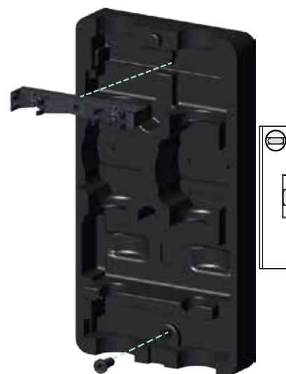
Abb. 7: Unterschale anschrauben
