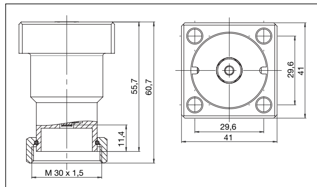
Maße
