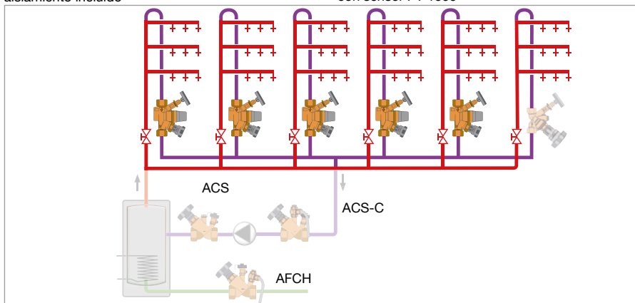
Sistema de circulación con “Aquastrum T plus” y “Aquastrum C”
