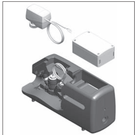
Abb. 3.1 Lieferumfang
