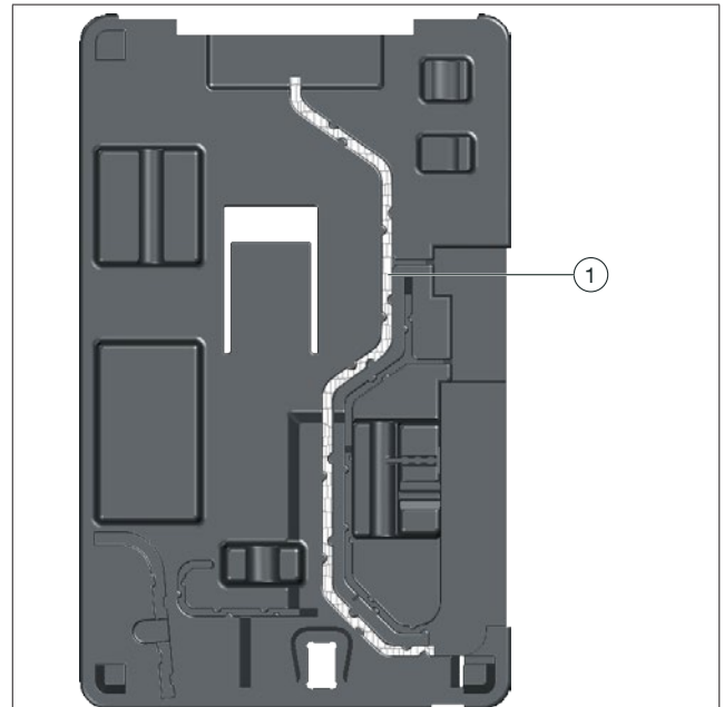
Abb. 13: Kabelführung
