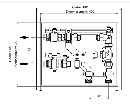
Illustr. 3.1.: Encombrenments raccordement latéral
