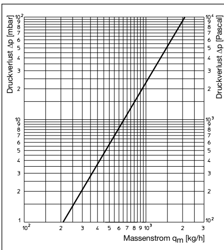
Abb. 7.1: Druckverlust „Floorbox“
