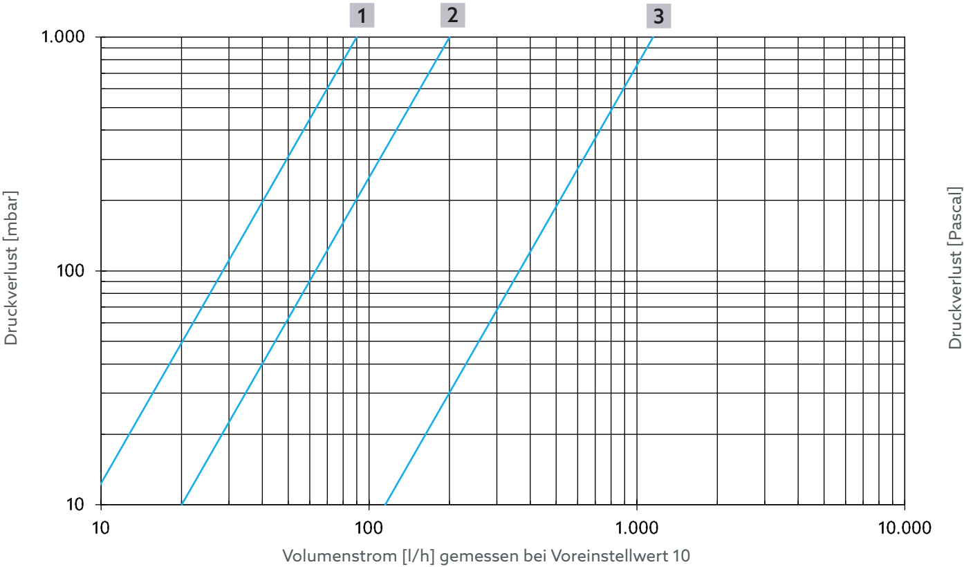
Abb. 17: Volumenstrom Thermische Regelung für Artikelnummer 4202504, 4202604, 4202704, 4202804
