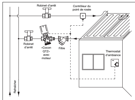
Illustr. 6.1 Système à deux tuyaux
