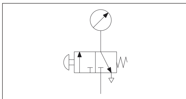
Schaltschema
