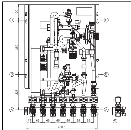
Abb. 5.1 Anschlussschema Kugelhahnansschlussleiste 1341080
