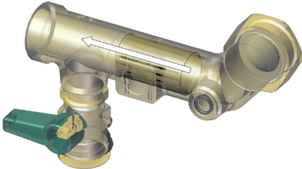
Abb. 37: Messturbine lösen
