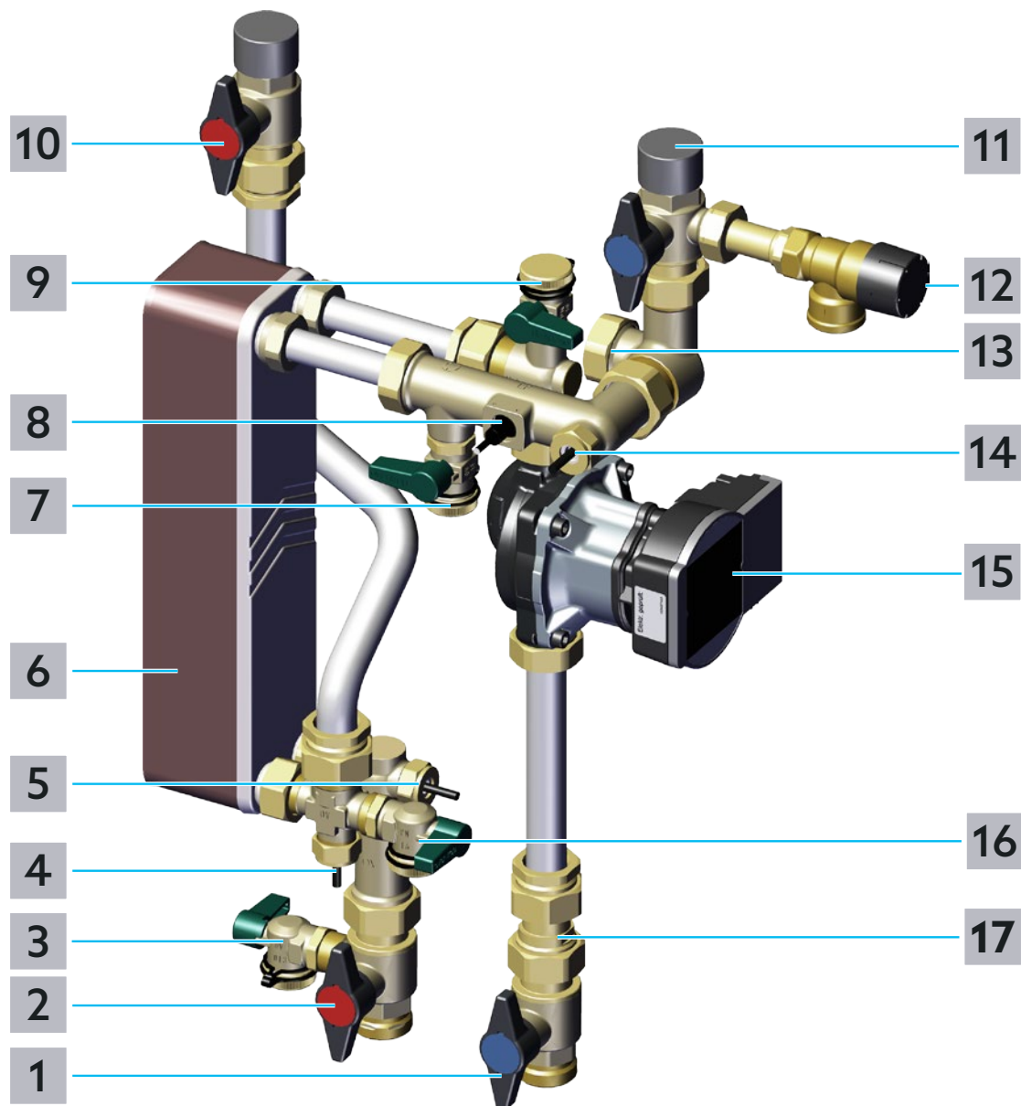
Abb. 2: Aufbau Armaturengruppe
