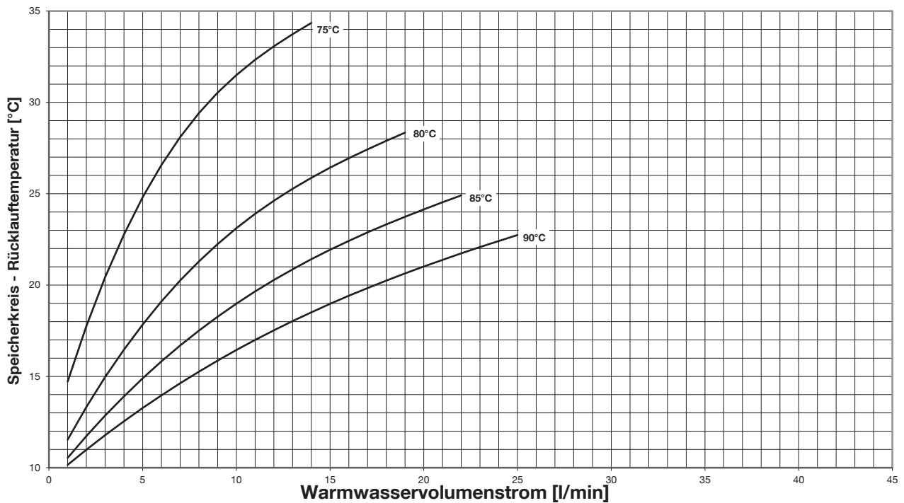
Abb. 55: Rücklauftemperatur Speicherkreis - Trinkwassererwärmung auf 75 °C
