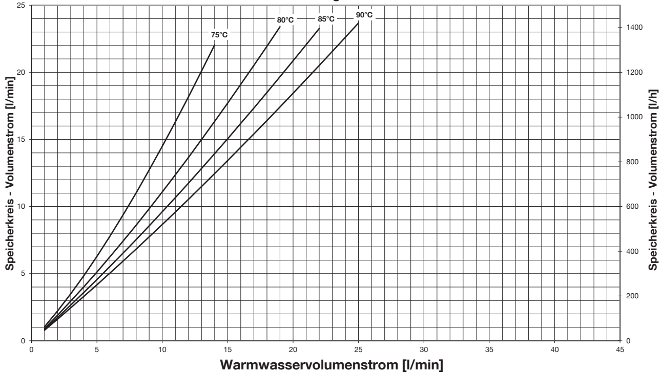
Abb. 54: Volumenstrom Speicherkreis - Trinkwassererwärmung auf 75 °C
