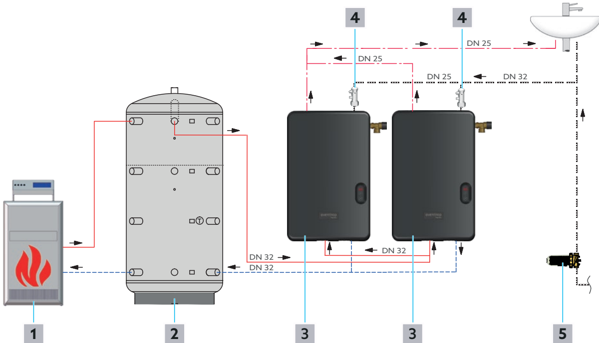
Abb. 4: Anlagenschema mit einem Speicher und zwei Frischwasserstationen
