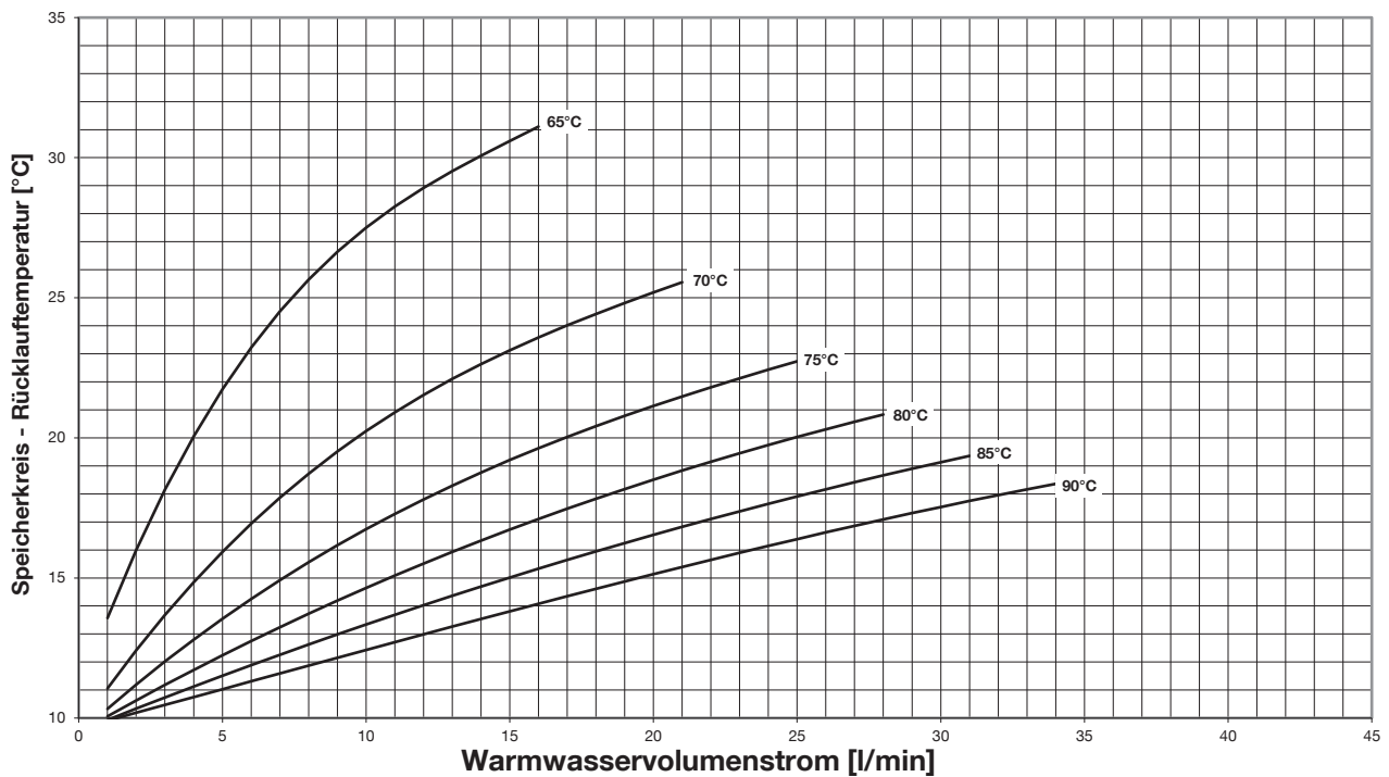
Abb. 51: Rücklauftemperatur Speicherkreis - Trinkwassererwärmung auf 65 °C
