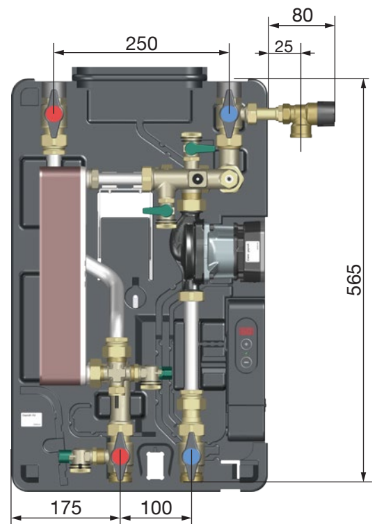
Abb. 6: Abmessungen Regumaq X-25 Unterschale mit Armaturengruppe
