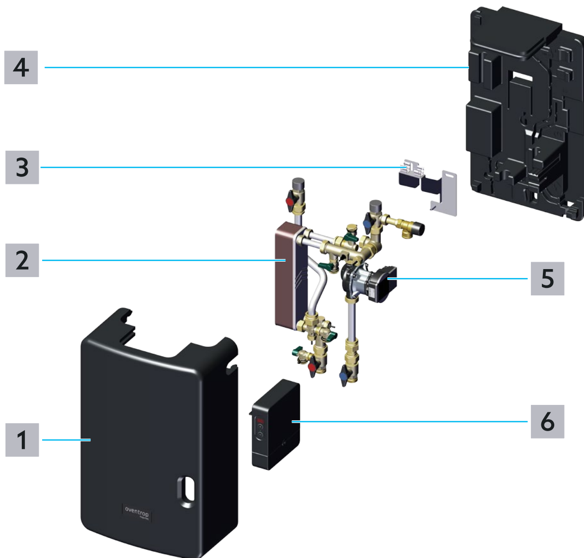
Abb. 1: Aufbau Station
