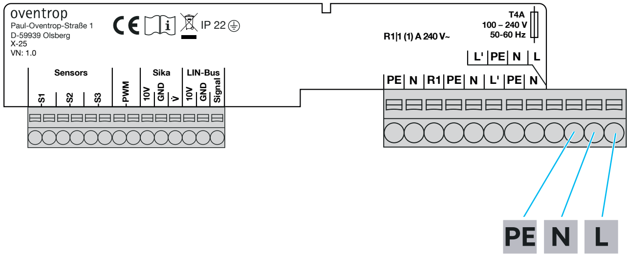
Abb. 9: Klemmbelegung
