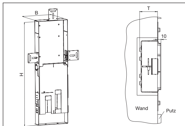
Übersicht Montagekanal
