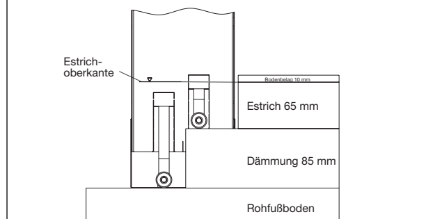
Maße bei maximaler Einbauhöhe von H = 490 \text{ mm} , Bügel komplett ausgefahren
