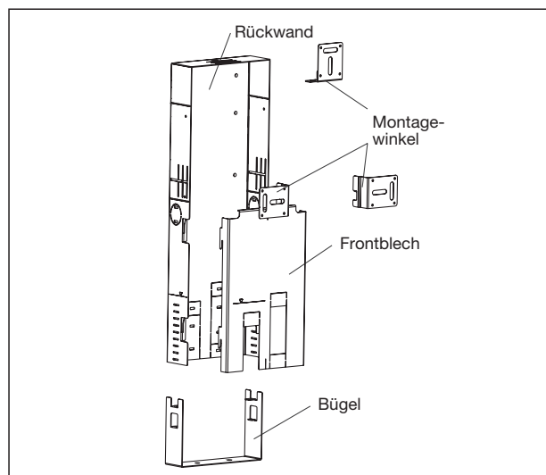
Übersicht Montagekanal
