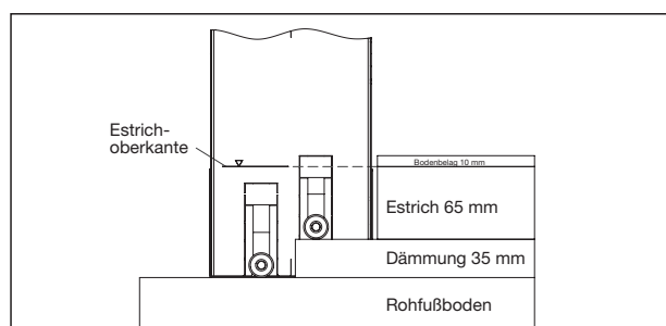
Maße bei minimaler Einbauhöhe von H = 440 \text{ mm} , Bügel komplett eingefahren
