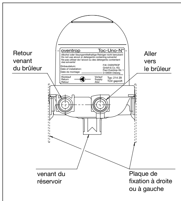
Vue côté brûleur:
