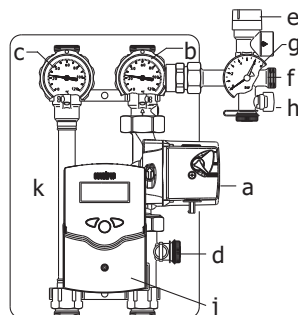
Фиг.: регулатор OV-„Regtronic BS/2“
