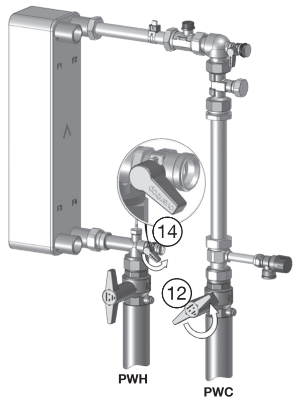
Abb. 4.17: Trinkwasser kalt (PWC) einleiten
