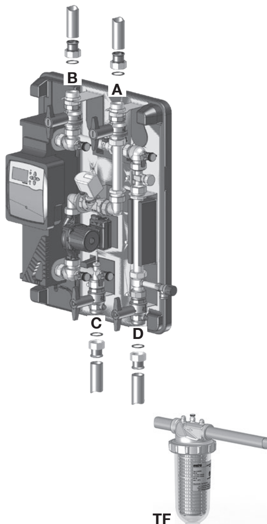
Abb. 4.8: Rohrleitungen mit Trinkwasser-Filter an Station anschließen
