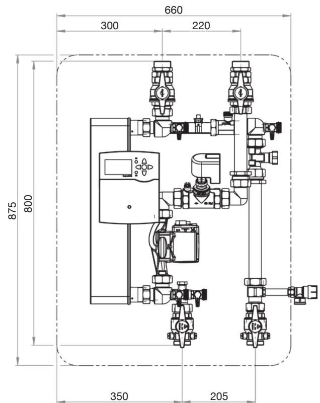
Abb. 3.8: Abmessungen „Regumaq X-70“ (Front)
