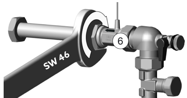
Abb. 5.16: Überwurfmuttern Volumenstromsensor lösen
