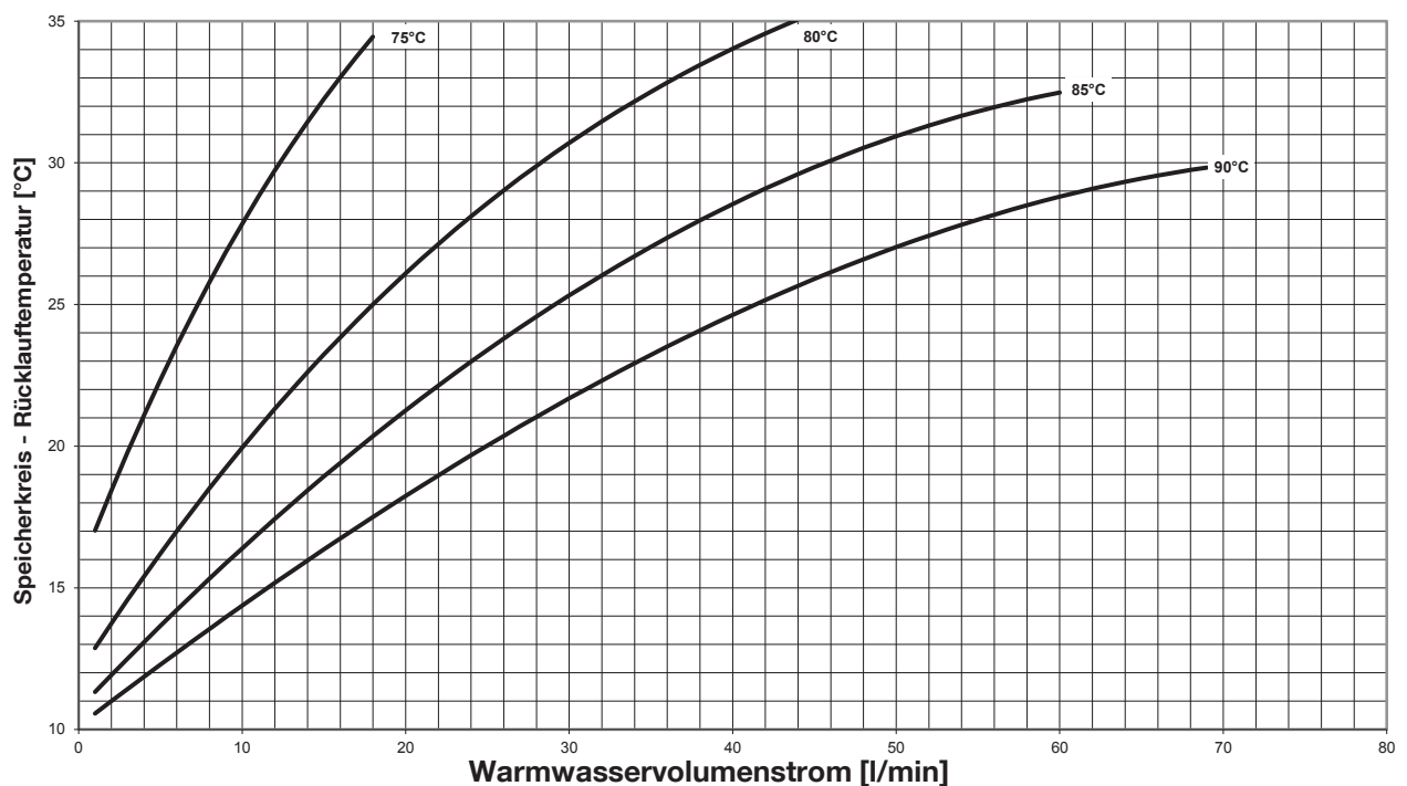
Rücklauftemperatur Speicherkreis bei unterschiedlichen Vorlauftemperaturen - Trinkwassererwärmung von 10 °C auf 75 °C -
