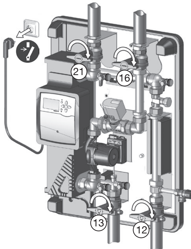
Abb. 5.13: Regler freischalten und alle Absperrkugelhähne schließen
