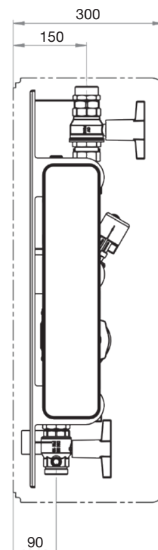
Abb. 3.9: Abmessungen „Regumaq X-70“ (Seite)
