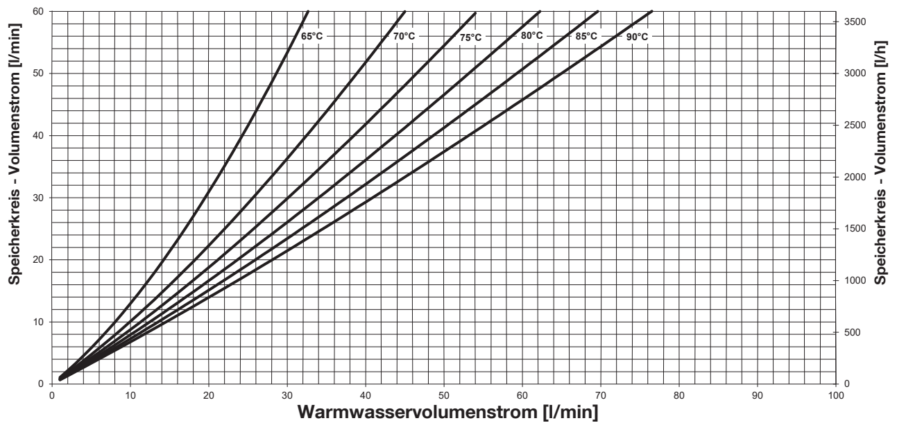
Rücklauftemperatur Speicherkreis bei unterschiedlichen Vorlauftemperaturen - Trinkwassererwärmung von 10 °C auf 65 °C -
