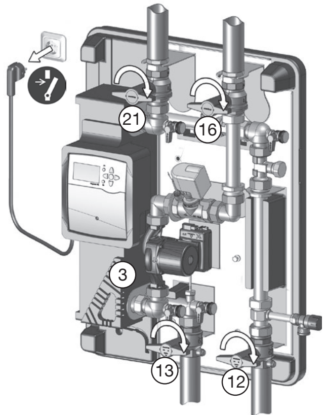
Abb. 5.1: Regler freischalten und Kugelhähne absperren
