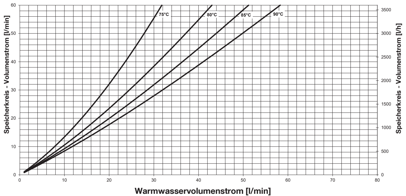
Rücklauftemperatur Speicherkreis bei unterschiedlichen Vorlauftemperaturen - Trinkwassererwärmung von 10 °C auf 75 °C -
