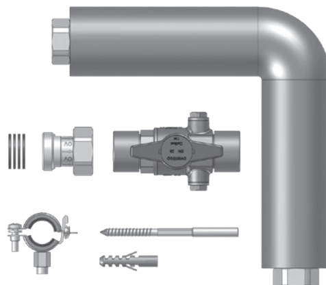
Abb. 3.10: Trinkwasser-Zirkulationsset, Art.-Nr. 1381590
