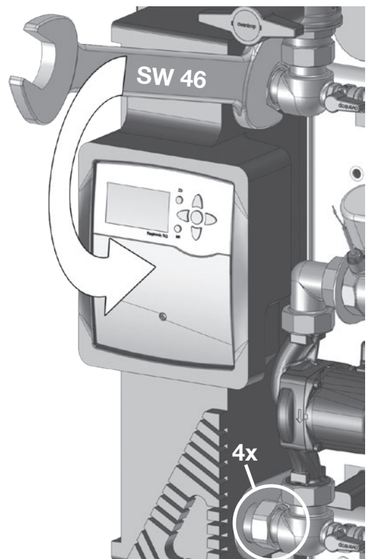
Abb. 5.6: Überwurfmutter des Wärmeübertragers lösen
