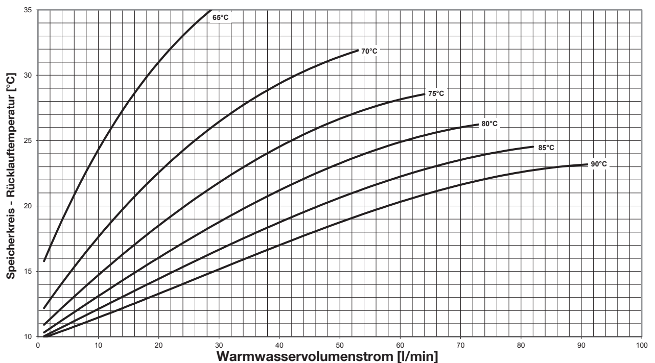
Rücklauftemperatur Speicherkreis bei unterschiedlichen Vorlauftemperaturen - Trinkwassererwärmung von 10 °C auf 65 °C -
