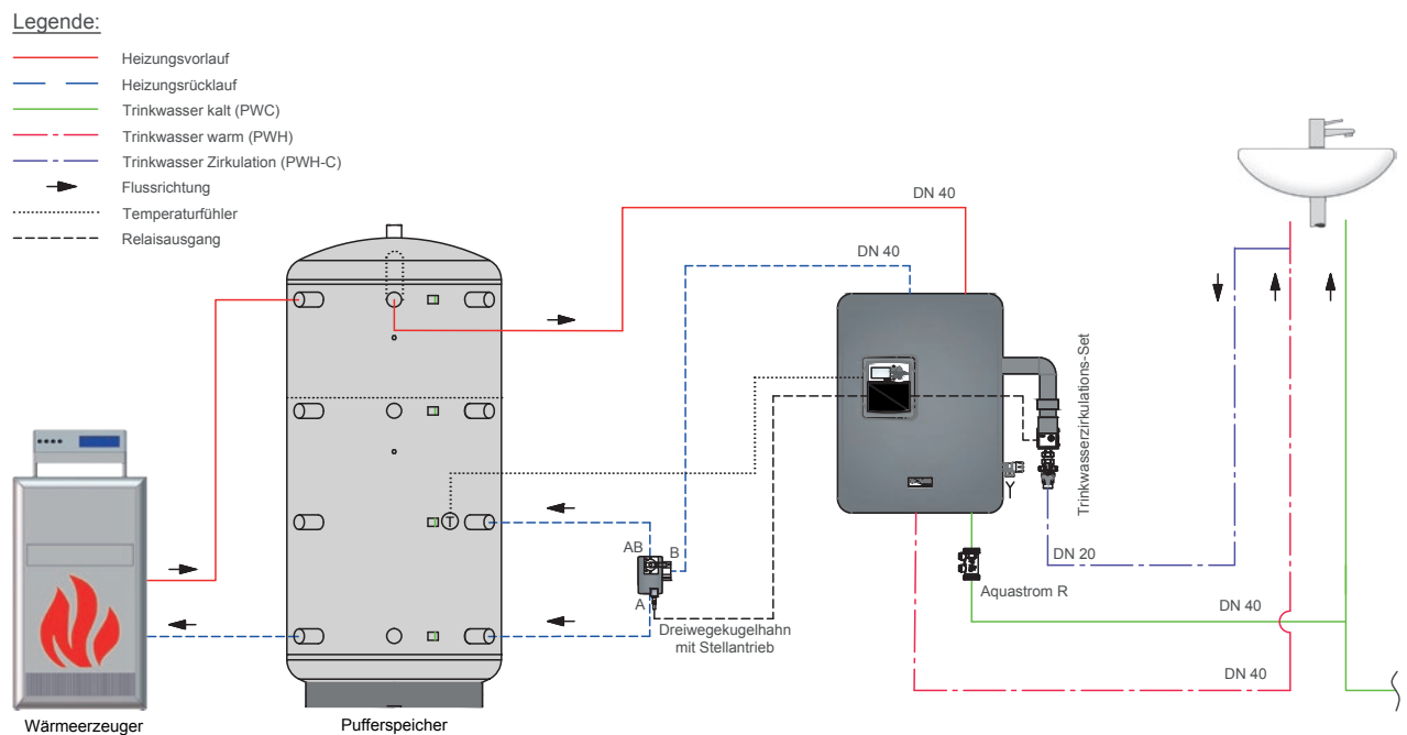
Abb. 3.5: Anlagenschema mit einer Frischwasser-Station „Regumaq X-70“
