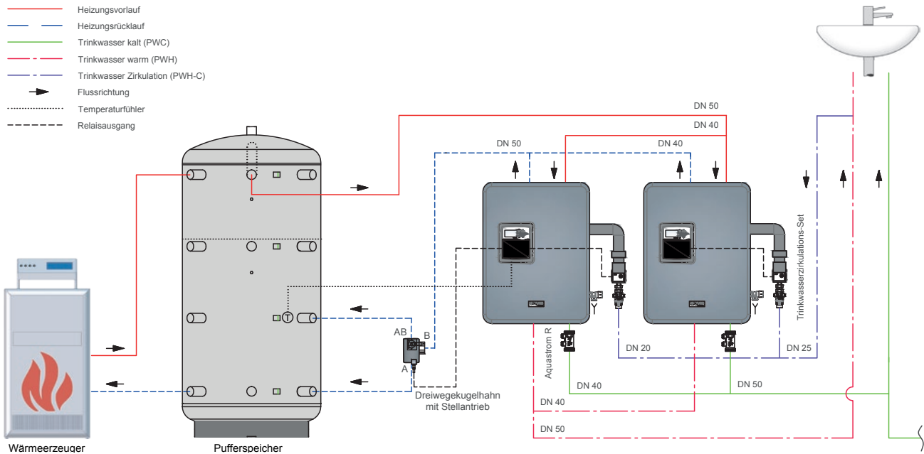
Abb. 3.6: Anlagenschema mit zwei Frischwasser-Stationen „Regumaq X-70“ („Tichelmann-System“)
