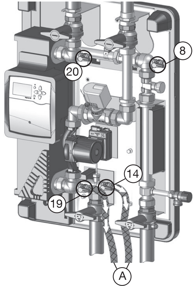
Abb. 5.5: Leitungen und Wärmeübertrager entleeren
