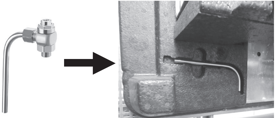
Abb. 3.13: Probeentnahmeventil (Art.-Nr. 4209102), kann während Nicht-Gebrauch in EPP-Unterschale eingesetzt werden
