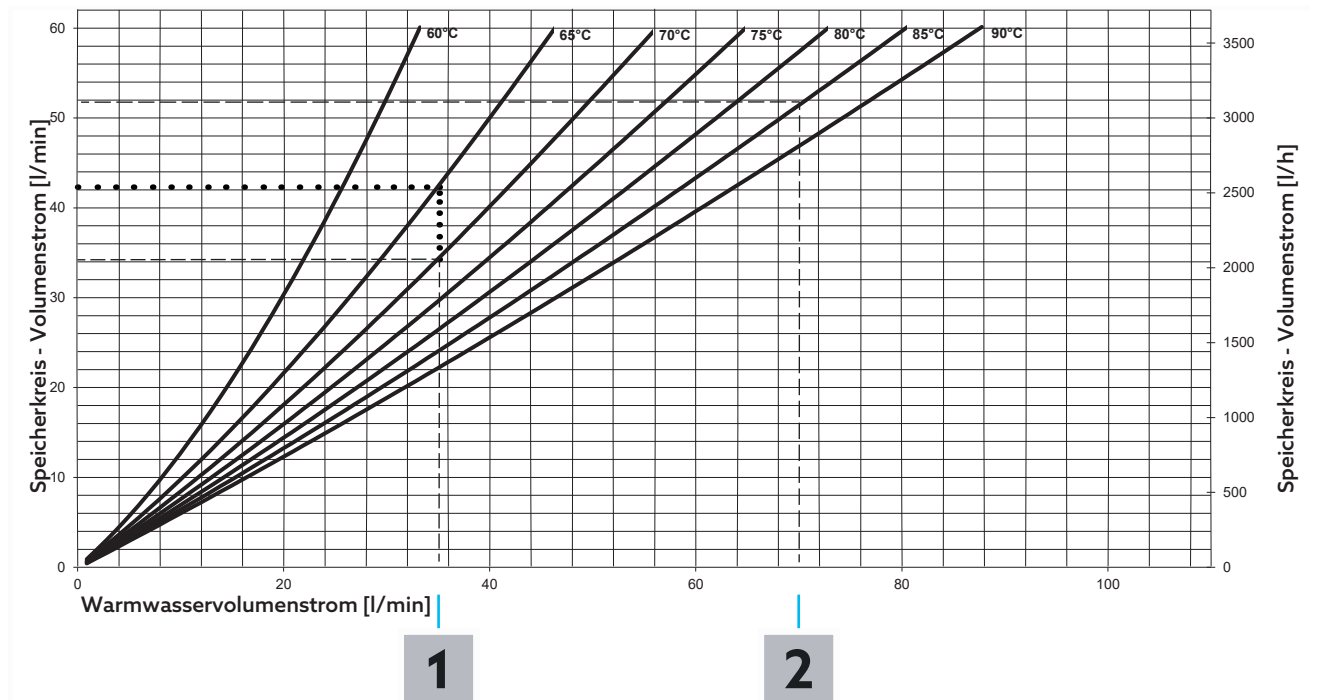
Abb. 3.4: Typischer Anwendungsfall „Trinkwassererwärmung 10 °C auf 60 °C“ (max. Zapfleistung von 70 l/min)*
