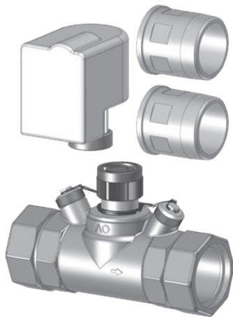
Abb. 3.14: Absperreinheit zur Verhinderung von Schwerkraftzirkulation, Art.-Nr. 1381078
