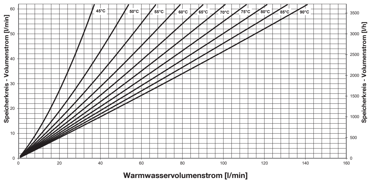
Rücklauftemperatur Speicherkreis bei unterschiedlichen Vorlauftemperaturen - Trinkwassererwärmung von 10 °C auf 45 °C -
