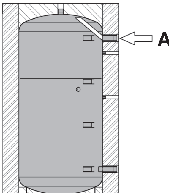
Abb. 4.7: Anschlussposition am Pufferspeicher für die Speicherkreis-Vorlaufzuleitung der Frischwasser-Station
