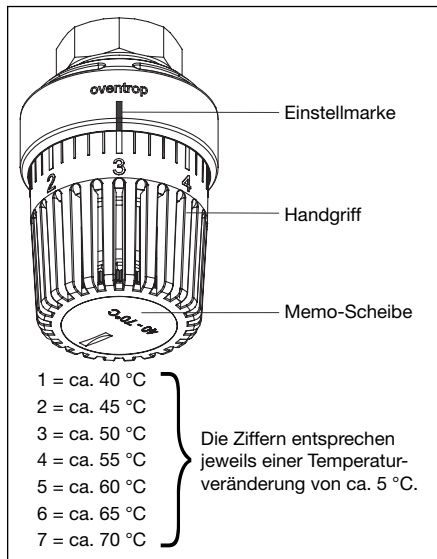
Abb. 8.4 Einstellung Trinkwassertemperatur
