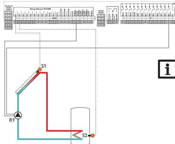
Пример электрического подключения высокоэффективного насоса
