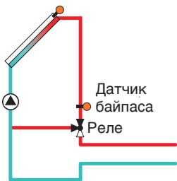
Примерная схема различных вариантов байпаса
