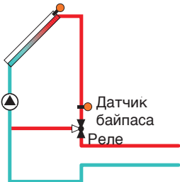
Вариант Клапан (обратное включение):
