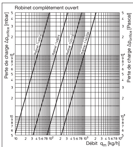
Diagramme 4.1 Débit en fonction de la perte de charge ( \Delta p_{\text{orifice}} ) par l'intermédiaire des prises de pression (voir fig. 4.1)
