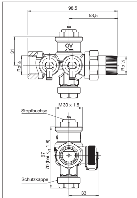
Abb. 4.2 Abmessungen
