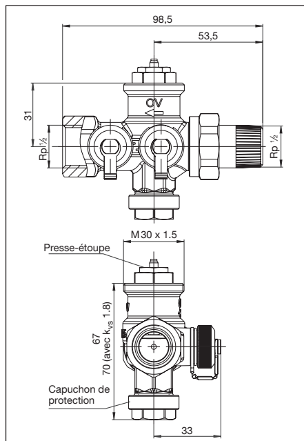
Fig. 4.2 Dimensions
