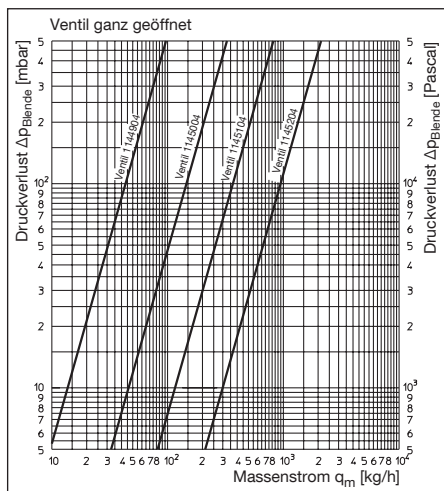
Diagramm 4.1 Durchfluss in Abhängigkeit vom Druckverlust ( \Delta p_{\text{Blende}} ) über die Messventile (siehe Abb. 4.1)
