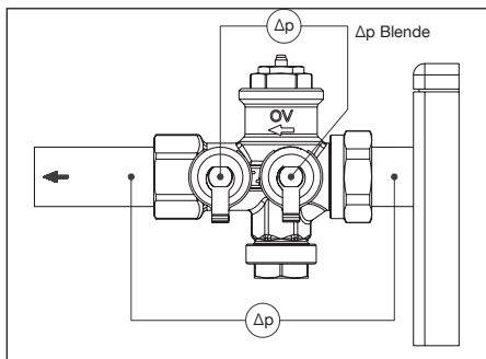
Abb. 4.1 Differenzdruckmessung
