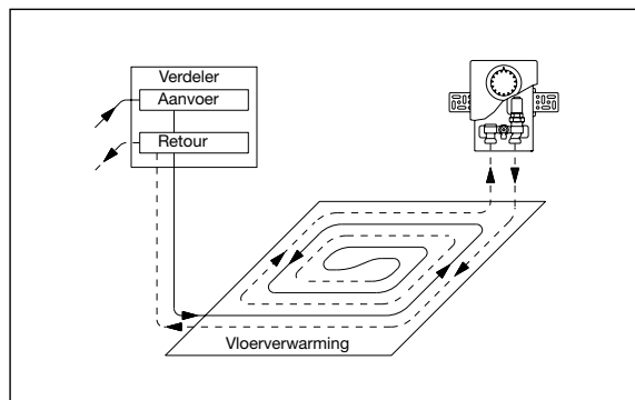
Montageschema temperatuurregeling per vertrek
