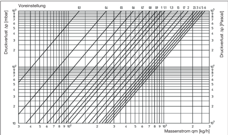
Diagramm 2: Druckverlust „Hycocoon VTZ“ Strangregulierungsventil DN 20
