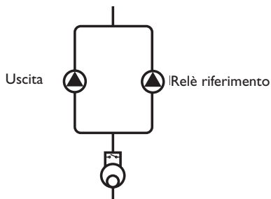
Schema esemplificativo di pompe accoppiate nella mandata solare con un flussometro a monte
