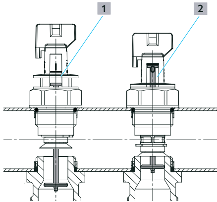
Fig. 5: Einstellung Durchflussindikator
