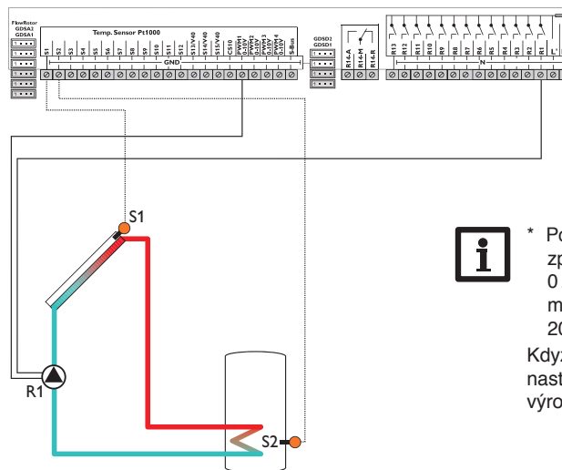
Příklad elektrického připojení vysoce účinného čerpadla
