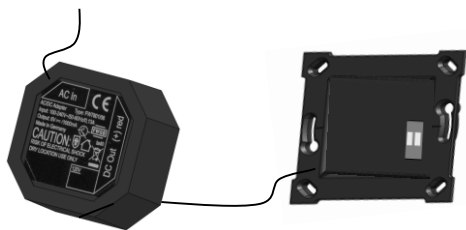
Bloc d'alimentation à encastrer avec fixation murale (Réf.: 1150692)
