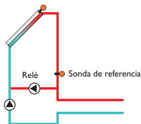
Variante con bomba:
