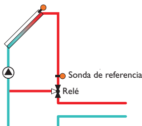
Variante con válvula (invertir):
