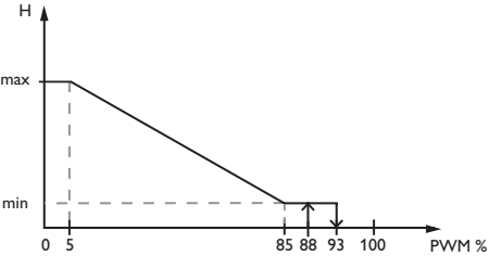
PWM D (por ejemplo fabricante WILO)
