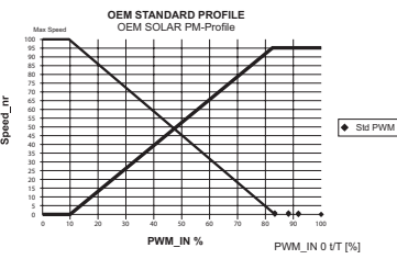
PWM E (por ejemplo fabricante Grundfos)
