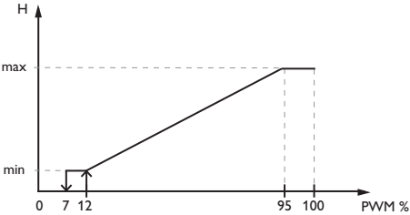
PWM A (por ejemplo fabricante WILO)
