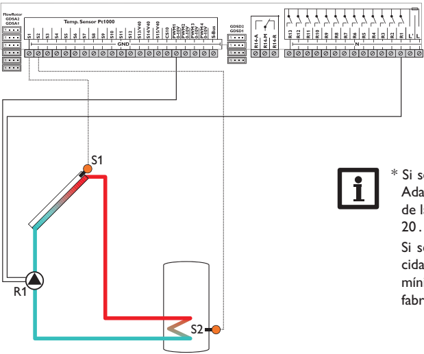
Ejemplo de conexión eléctrica de una bomba de alta eficiencia
