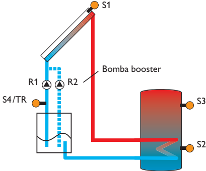
Figura de ejemplo de un sistema drainback (R2 = bomba de refuerzo (booster))
