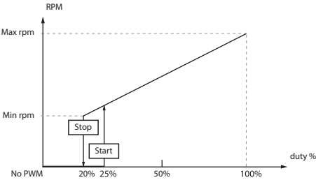
PWM C (por ejemplo fabricante Laing)
