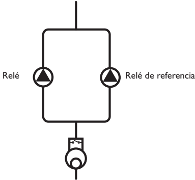
Figura de ejemplo de bombas paralelas en el avance solar con un caudalímetro aguas arriba
