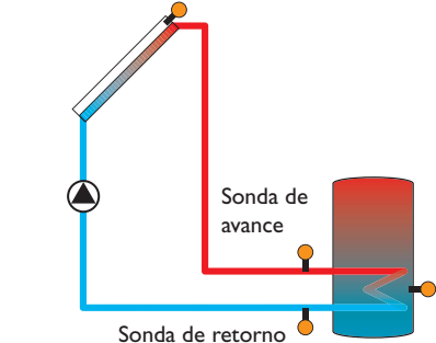
Ejemplo de posición de las sondas de avance y retorno
