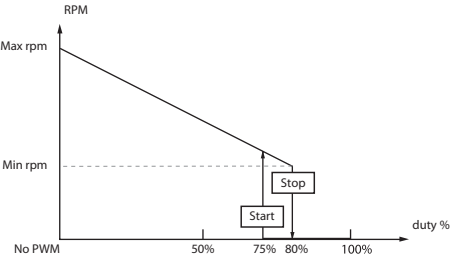
PWM F (por ejemplo fabricante Laing)
