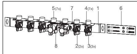
Fig. 3.1 Bloc de raccordement avec robinets à tournant sphérique
