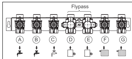
Abb. 5.1 Anschlusskennzeichnung
