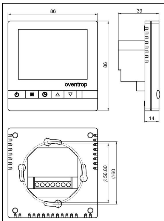
Abb. 4.1 Abmessungen
