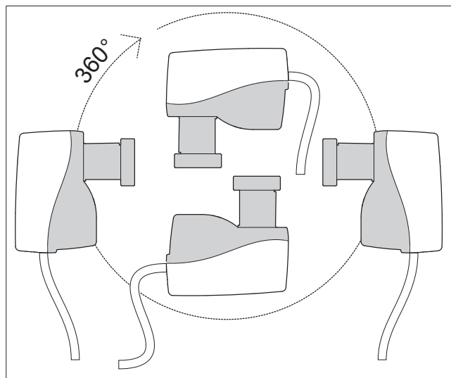
Abb. 3: Einbaulage
