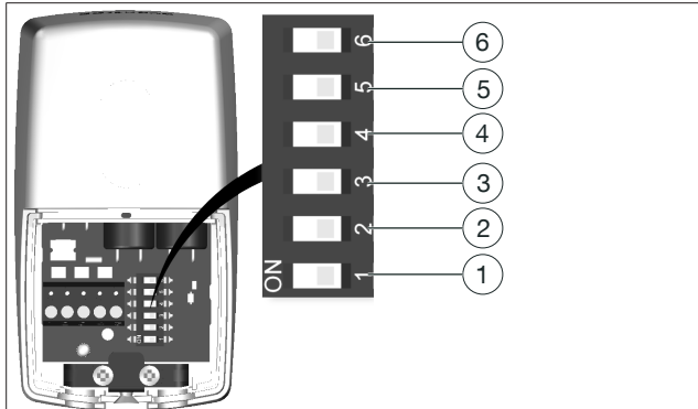
Abb. 4: DIP-Schalter
