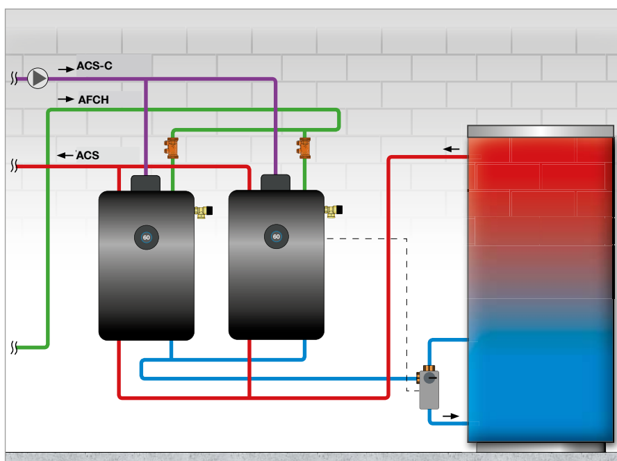
Conexión en cascada “Regumaq X-45”
