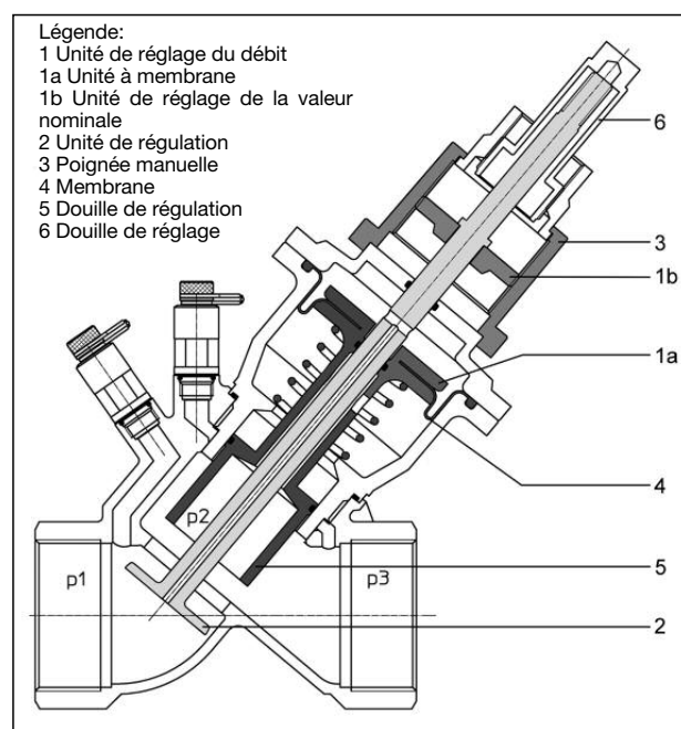
Fig. 5 Configuration du robinet «Cocon QTR»
