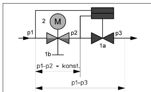
Fig. 6 Principe de fonctionnement du robinet «Cocon QTR»
