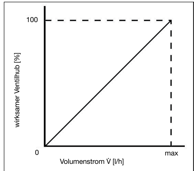
Abb. 9 Kennlinie des „Cocon QTR“ Ventils
