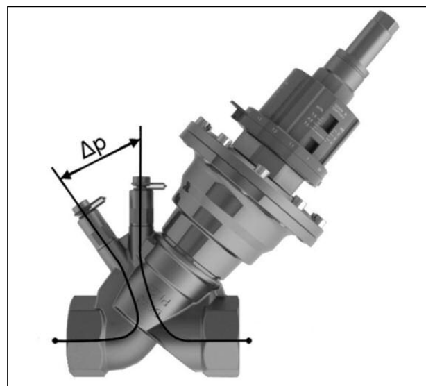
Fig. 4 Pression différentielle
