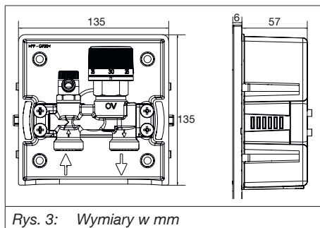
Rys. 3: Wymiary w mm
