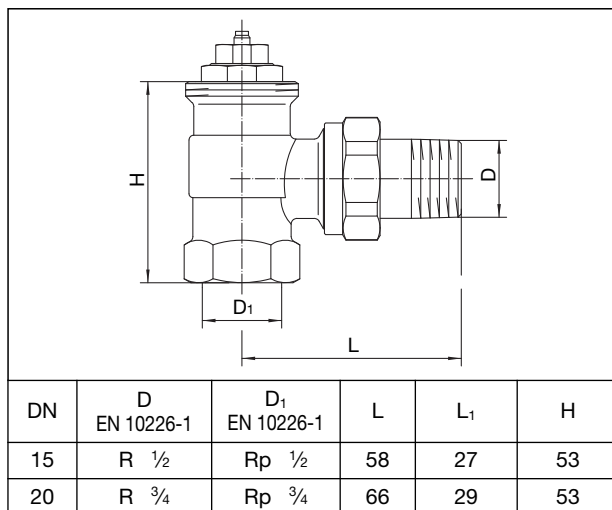
Dimensiuni ventil colțar
