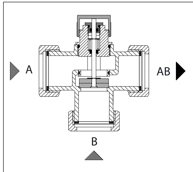
Schnittbild
