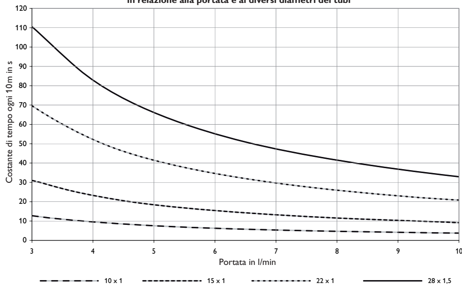
Costante di tempo \Delta t circ. ogni 10 m di tubazione in rame, in relazione alla portata e ai diversi diametri dei tubi
