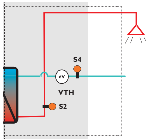
Circuito secondario
