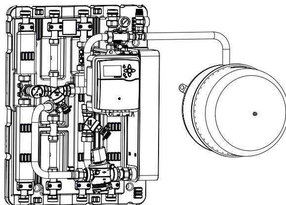
Fig. 40: Vase d'expansion à membrane monté
