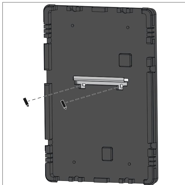
Fig. 27: Marquage des trous de perçage pour l'équerre de fixation
