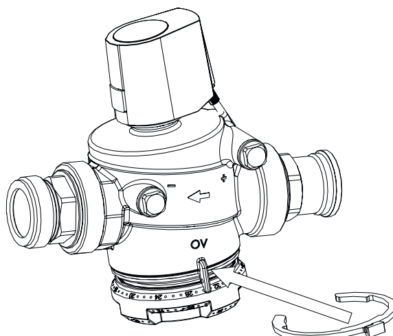
Fig. 47: Remontage du bague de blocage
