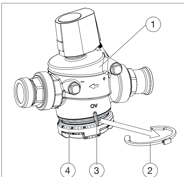
Fig. 45: Démontage du bague de blocage
