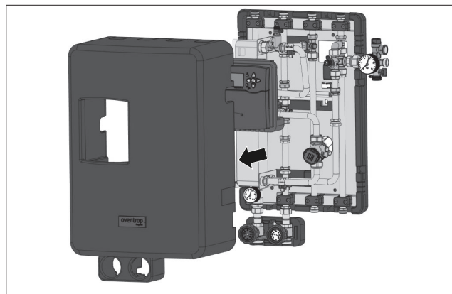
Fig. 26: Démontage de l'isolation avant
