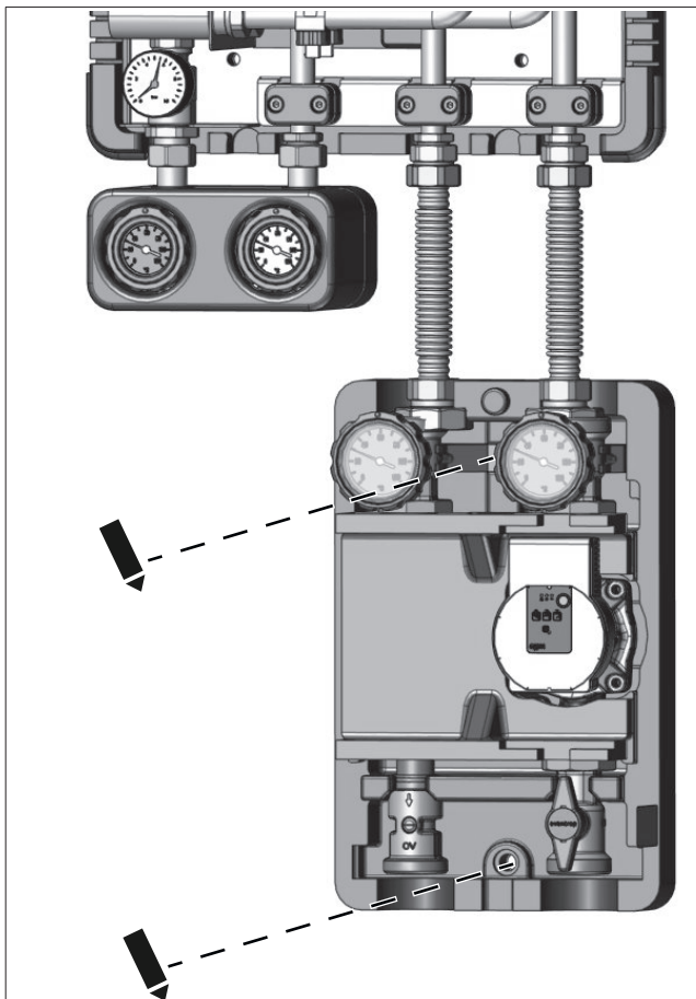
Fig. 31: Vissage du groupe avec circulateur (raccordement par le bas)
