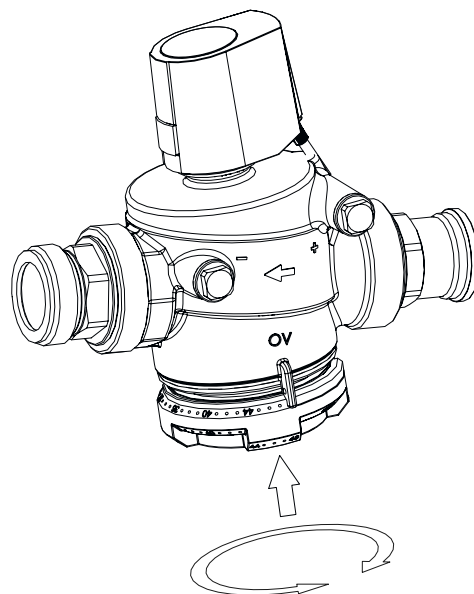
Fig. 46: Réglage de la valeur de consigne
