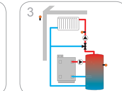
Смесен отоплителен кръг с допълнително отопление и зареждаща помпа
