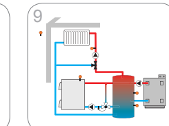
Смесен отоплителен кръг с котел на твърдо гориво и допълнително отопление
