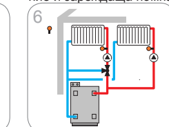
Смесен и несмесен отоплителен кръг
