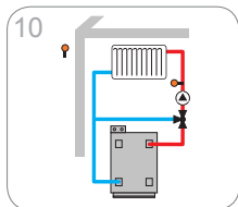
Смесен отоплителен кръг с централен външен сензор (Slave)
