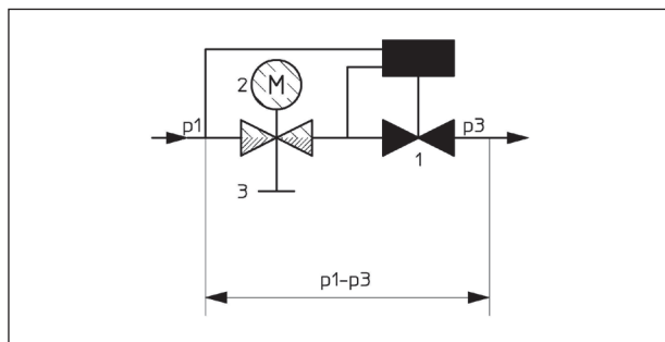
Pression différentielle
