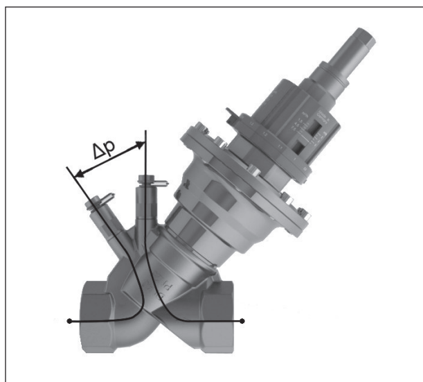
Pression différentielle
