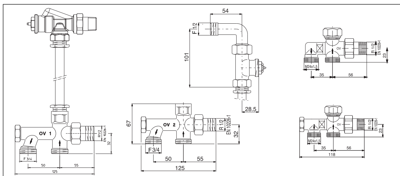
Dimensiuni „Bypass-Combi Uno/Duo”
