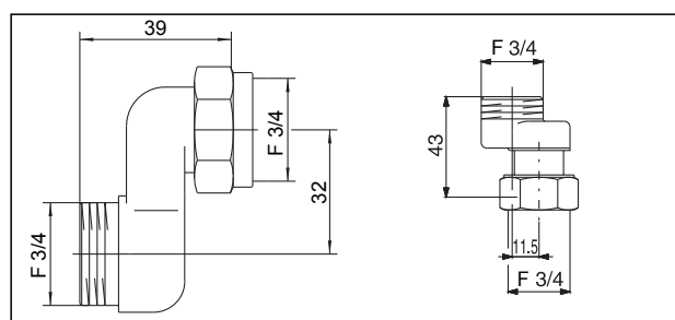
Dimensiuni racord de îmbinare cu filet S
