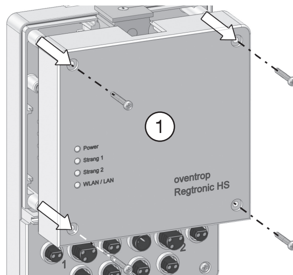
Abb. 39: Gehäusedeckel des Reglers abnehmen
