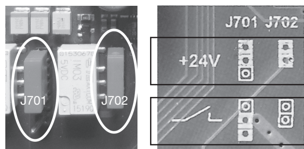
Abb. 40: Steckbare Jumper auf der Hauptplatine
