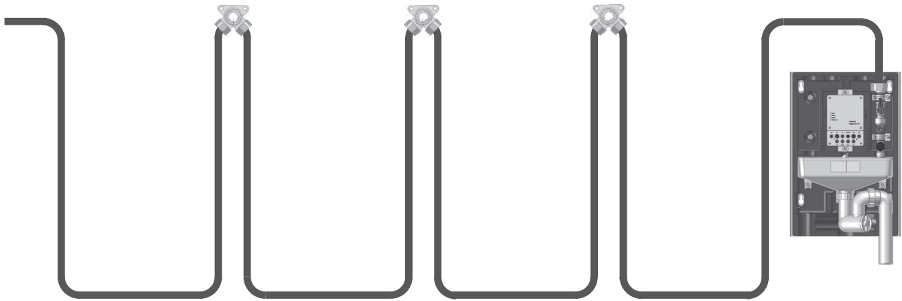
Spülstation „Regudrain Uno“ (1-Strang) an Reihenleitung (Beispiel)
