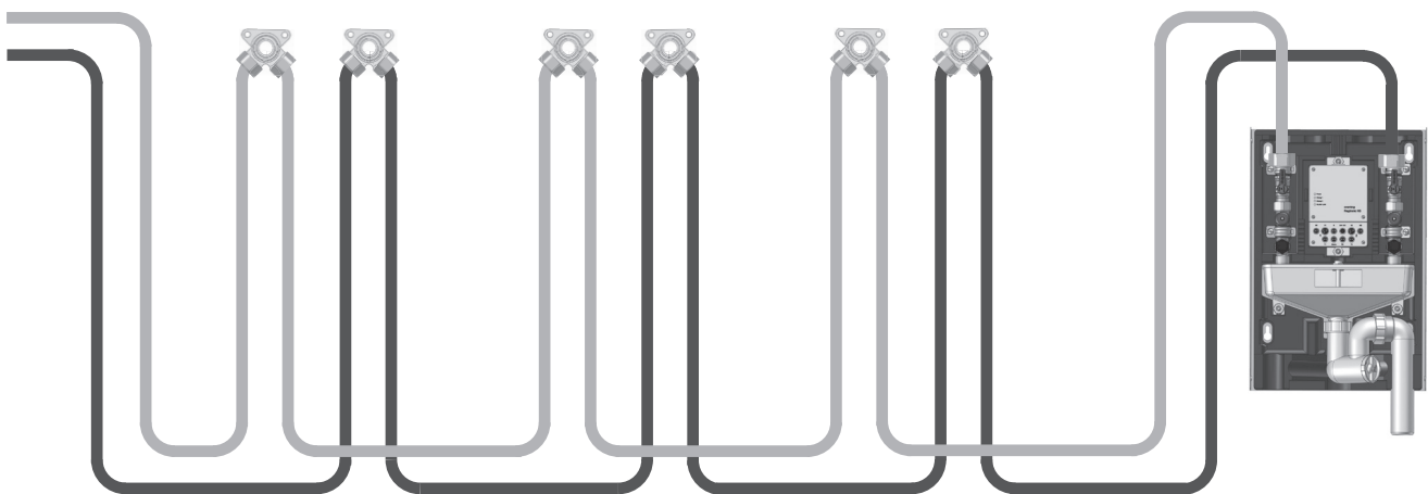
Spülstation „Regudrain Duo“ (2-Strang) an Reihenleitung (Beispiel)
