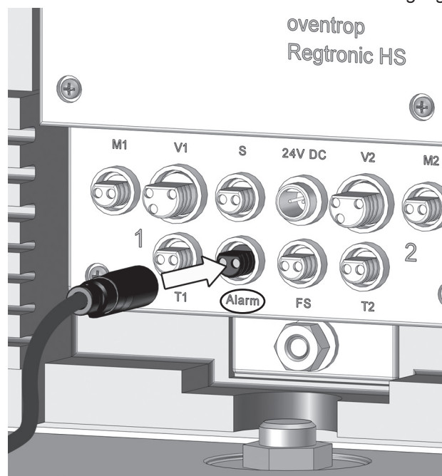
Abb. 38: Anschluss Sensorkabel an Alarmausgang
