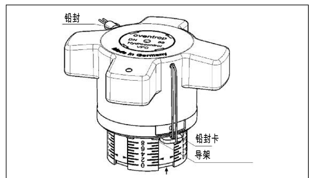
图7.2 手轮的锁定
