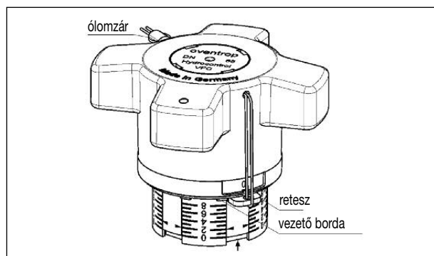
7.2 ábra. A kézikérék rögzítése
