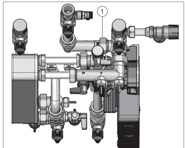
Abb. 7: Frischwasserstation incl. Zirkulationsset ohne Hocheffizienzpumpe
