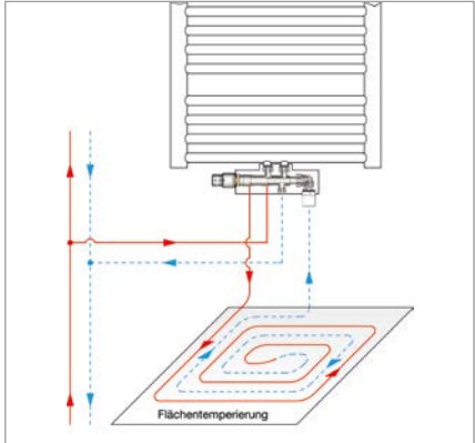
System-Darstellung „Multiblock T-RTL“ mit Flächentemperierung
