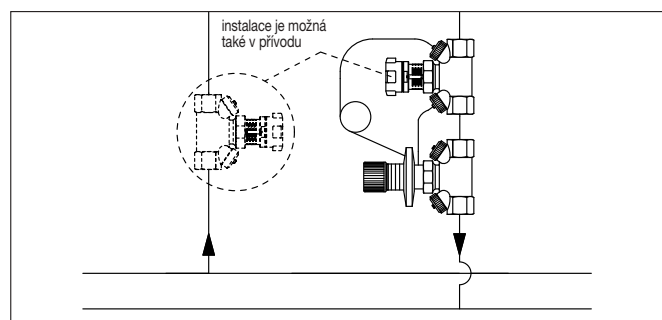
Příklad: Regulace průtoku pomocí kombinace armatur, regulátoru diferenčního tlaku „Hycococon DP“ a smyčkového regulačního ventilu „Hycococon V“
