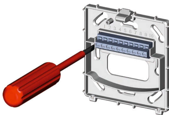
Fig. 9: ClimaCon F - Branchement électrique
