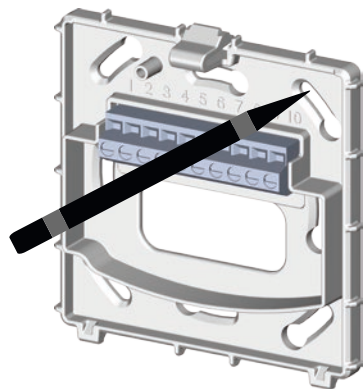
Fig. 8: Montage de la plaque de montage
