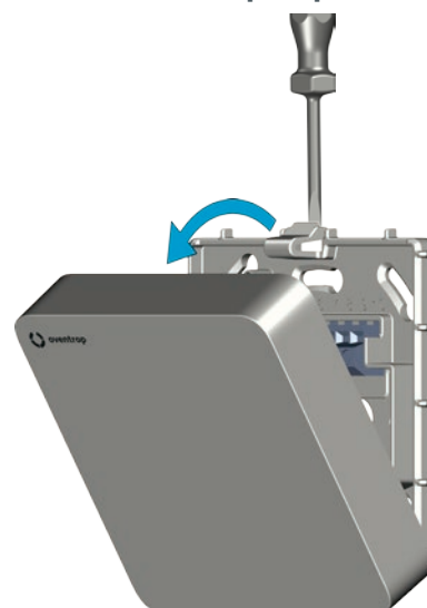
Fig. 7: Libération de la plaque de montage
