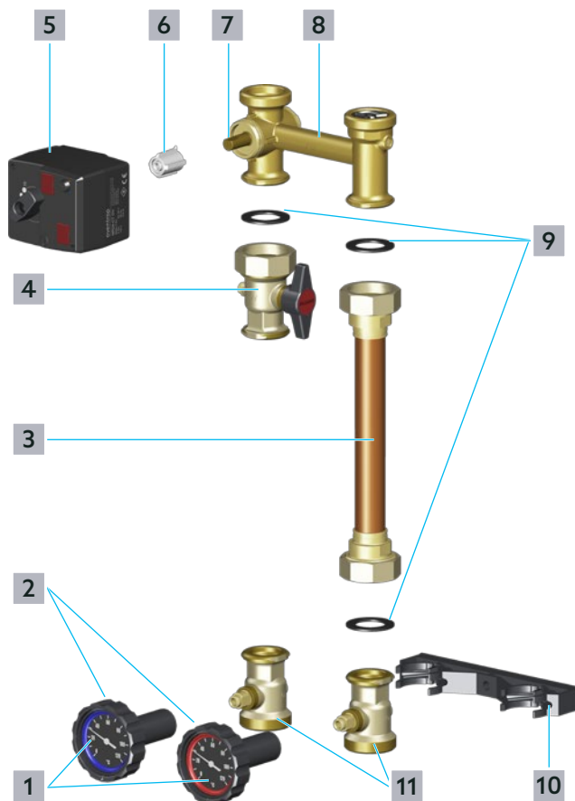
Abb. 2: Aufbau Armaturengruppe
