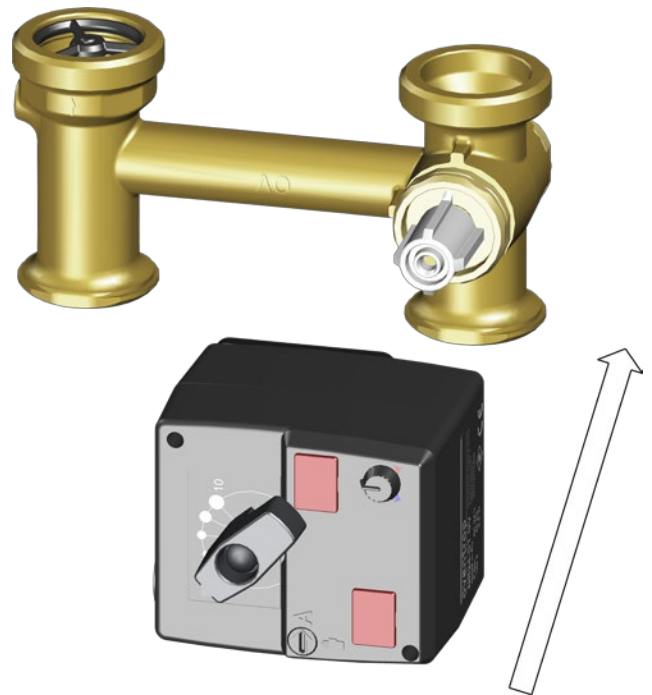
Abb. 39: Regler montieren
