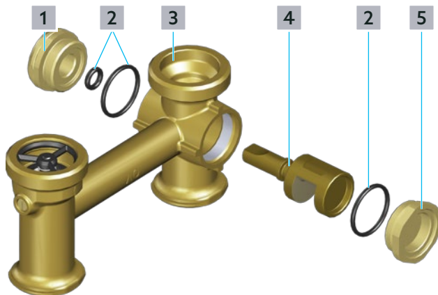
Abb. 34: Mischhahn Aufbau
