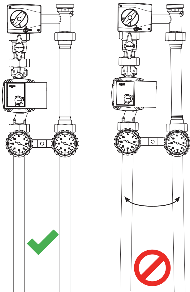
Abb. 25: Spannungsfrei verrohren
