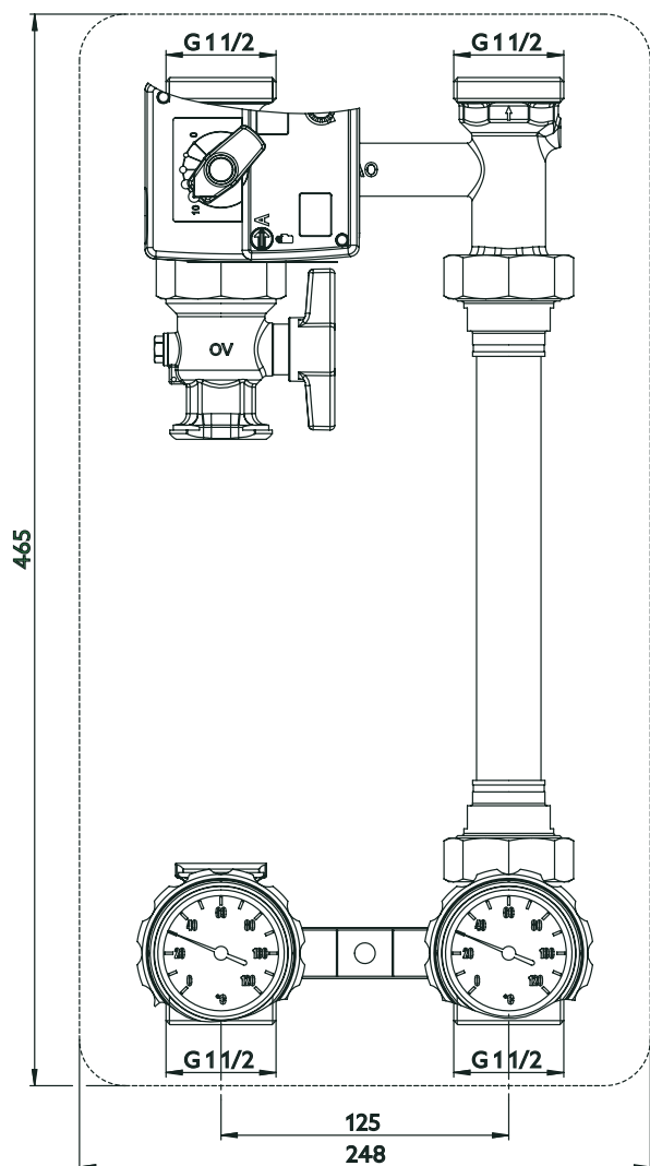
Abb. 20: Vorderansicht
