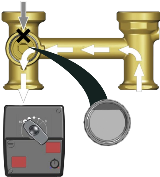
Abb. 15: Bypass Heizungs-Kreis vom Festbrennstoffkessel
