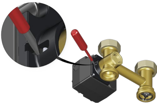
Abb. 30: Stellmotor vom Mischhahn abziehen
