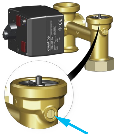
Abb. 19: Sperrventil geöffnet (Befüllung, Wartung)
