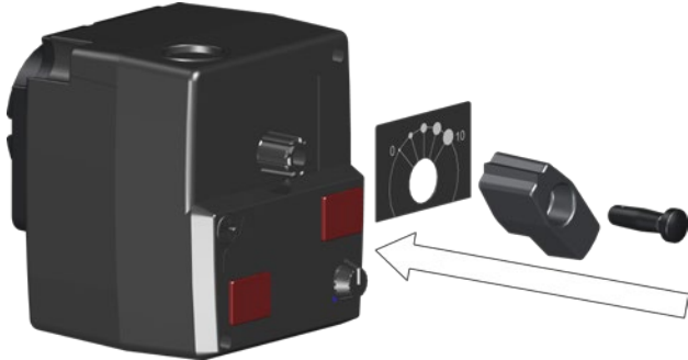
Abb. 33: Drehgriff montieren
