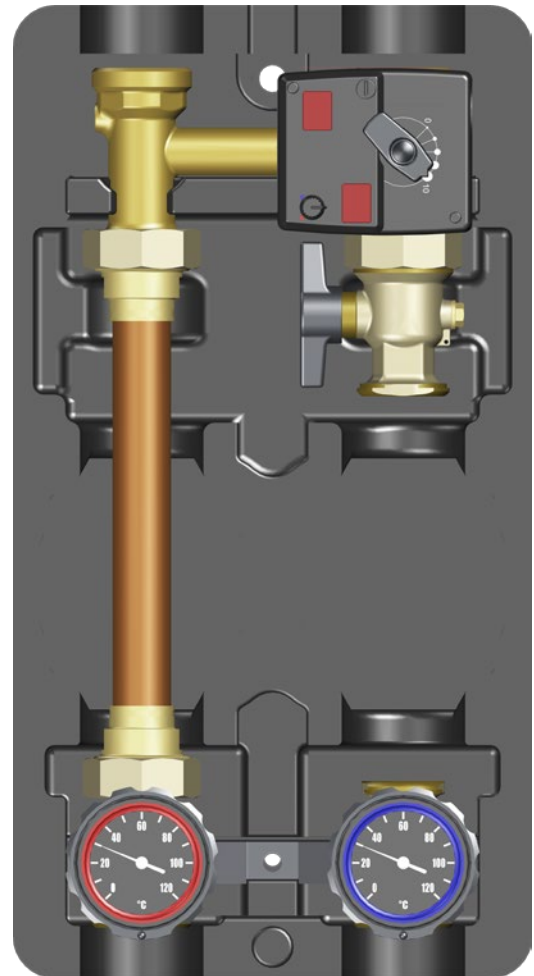
Abb. 28: Vorlaufstrang links
