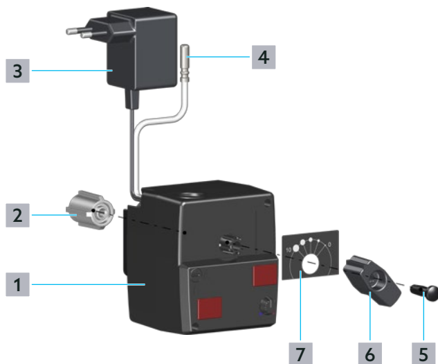
Abb. 3: Aufbau Stellmotor mit Festwertregelung
