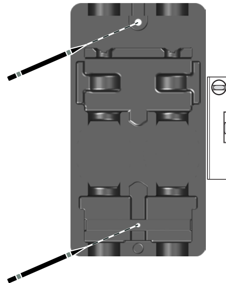
Abb. 22: Unterschale als Bohrschablone
