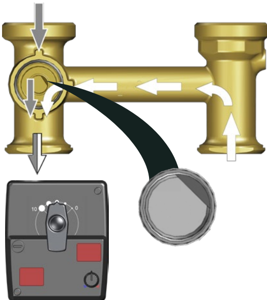
Abb. 16: Heizkreis teilweise geöffnet
