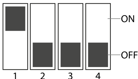
Abb. 5: DIP-Schalter Werkseinstellung
