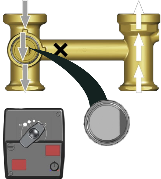
Abb. 17: Heizkreis vollständig geöffnet
