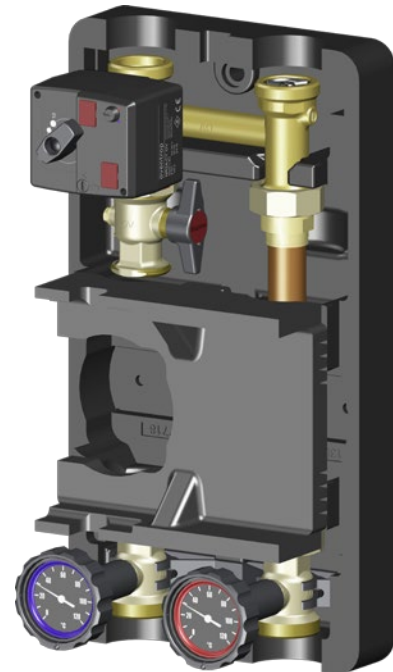
Abb. 24: Armaturengruppe eingehängt (Darstellung ohne Pumpe)
