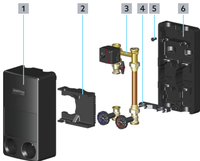
Abb. 1: Aufbau Station
