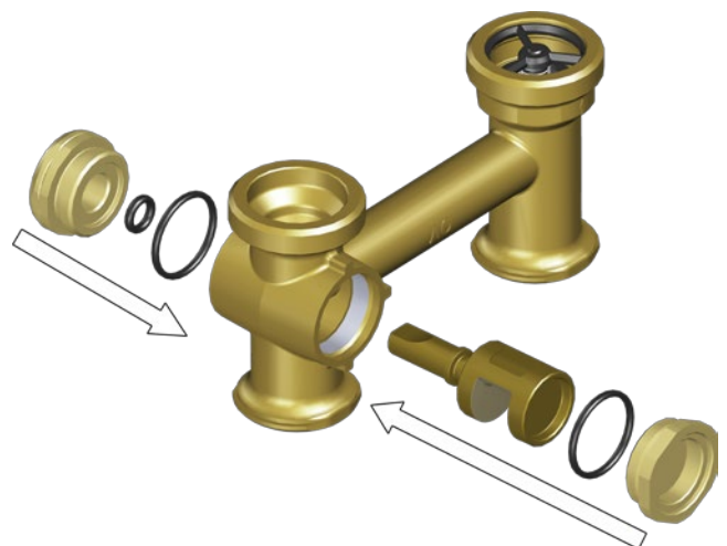
Abb. 36: Mischhahn montieren
