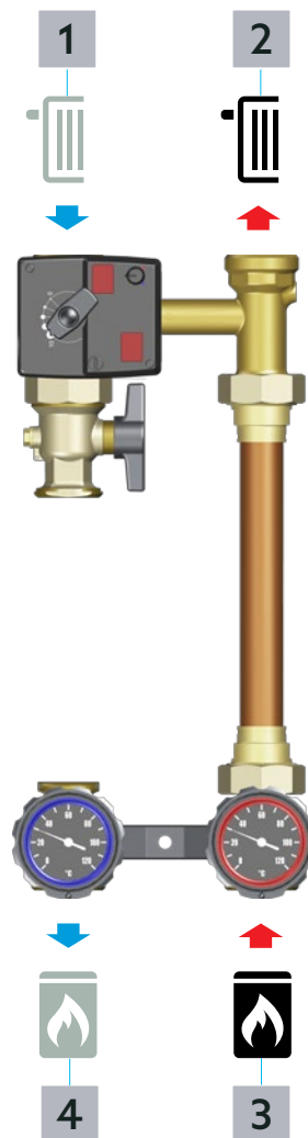
Abb. 26: Verrohrung (Darstellung ohne Pumpe)
