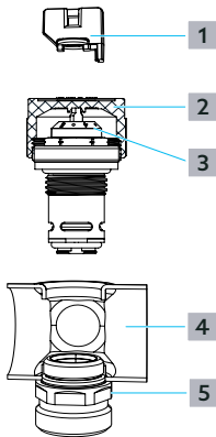
Fig. 3: Aufbau Ventileinsatz QM
