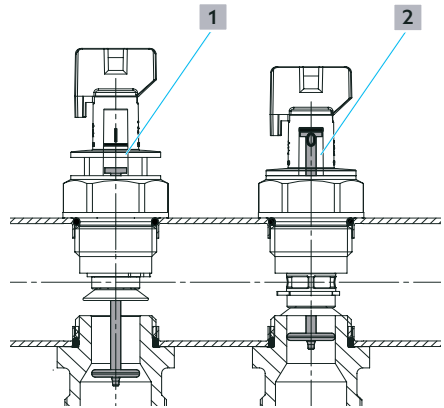
Fig. 5: Einstellung Durchflussindikator
